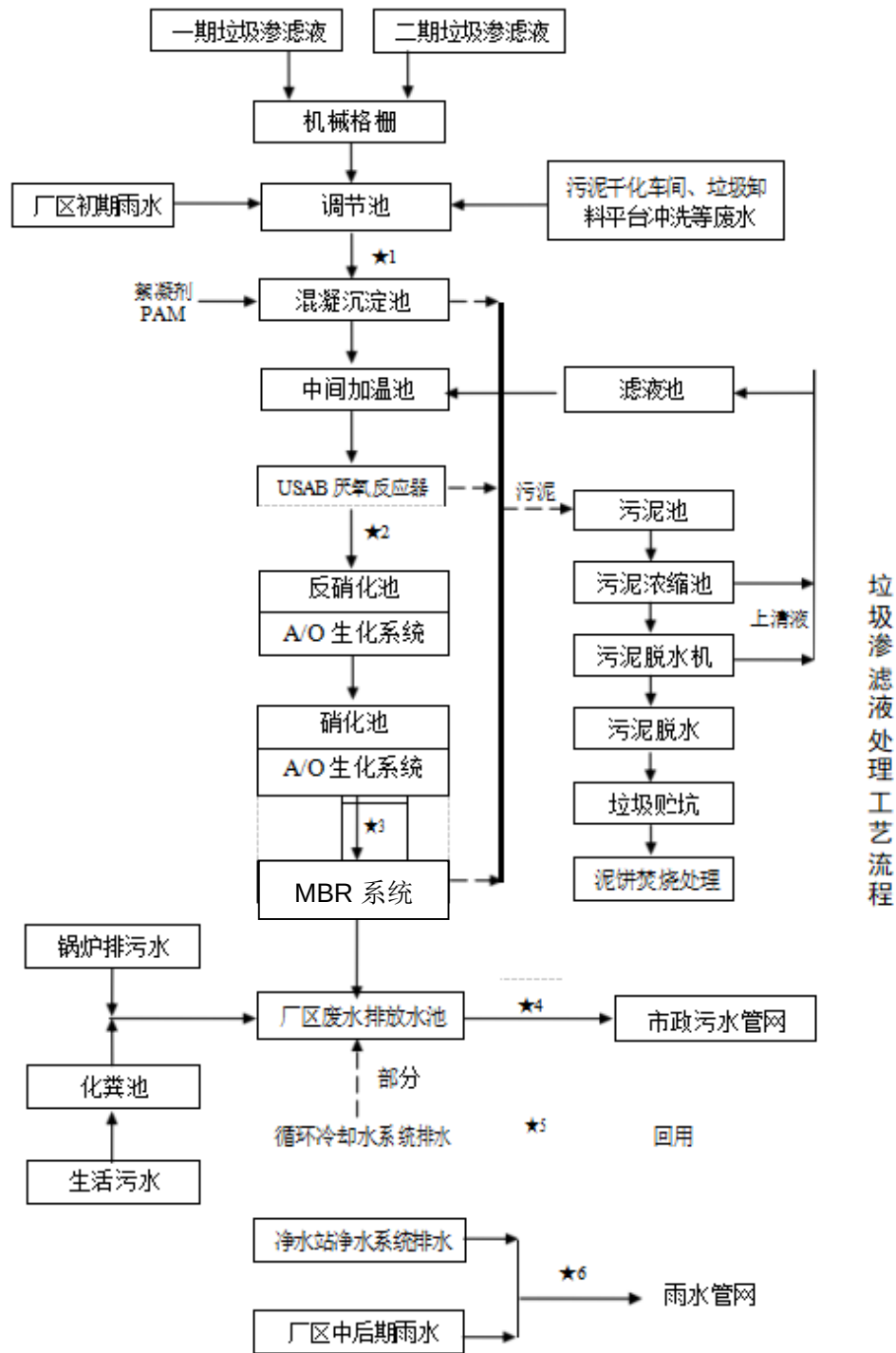
图 3-7 一期、二期项目污水处理设施流程图
