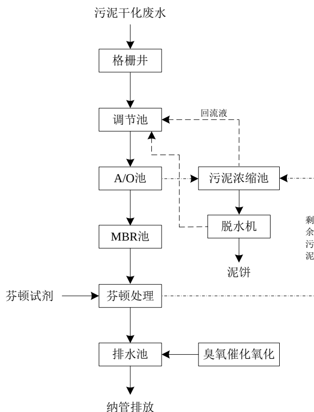
图 7-5 污泥干化项目污水处理设施流程图
