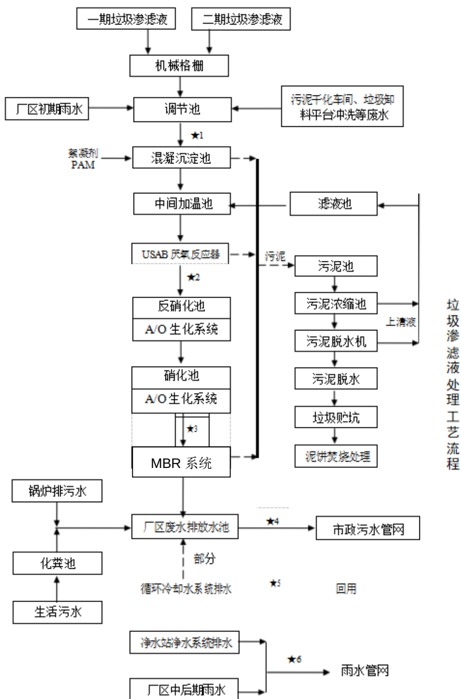
图 7-4 一期、二期项目污水处理设施流程图
