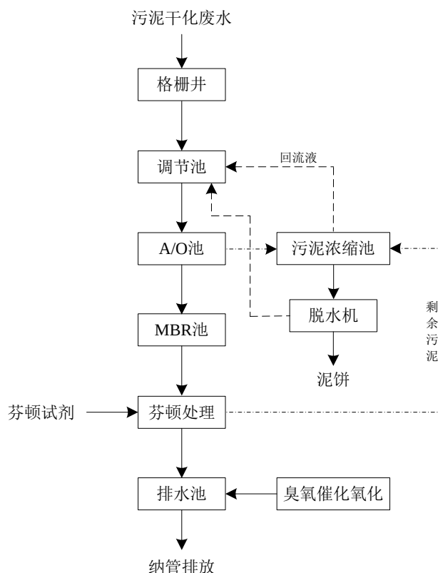
图 3-8 污泥干化项目污水处理设施流程图
