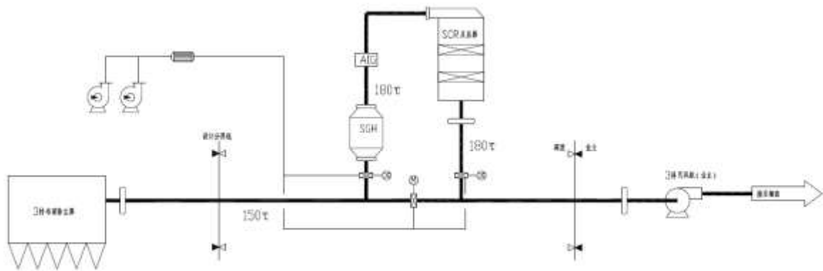
图 7-3 改造后低温 SCR 流程图
