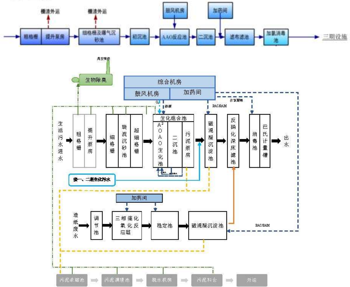
图 5-6 项目全厂污水处理工艺流程图
