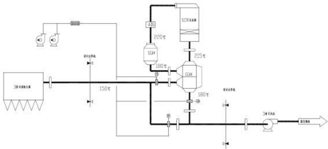
图 7-2 原二期中温 SCR 流程图
