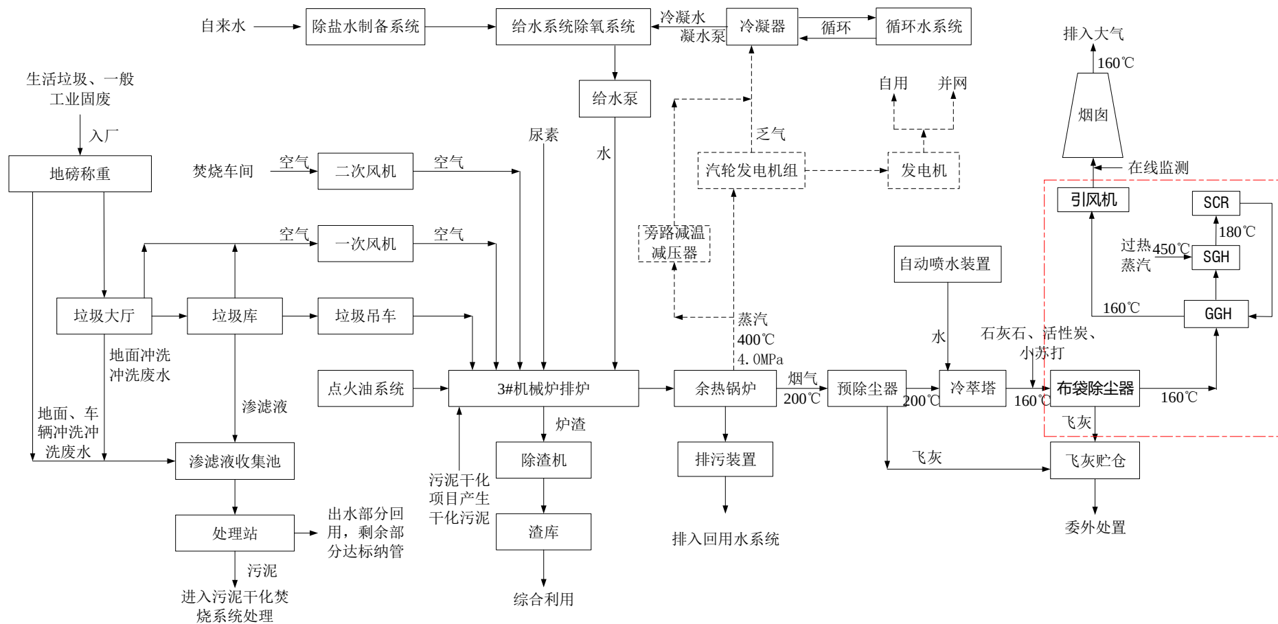
图 4-1 项目 3#炉生产工艺流程图
