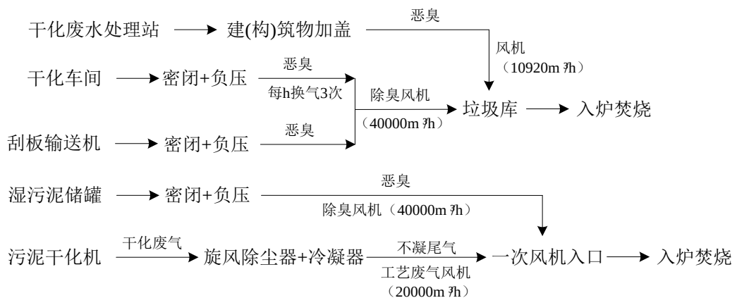
图 3-6 污泥干化项目废气处理设施流程图
