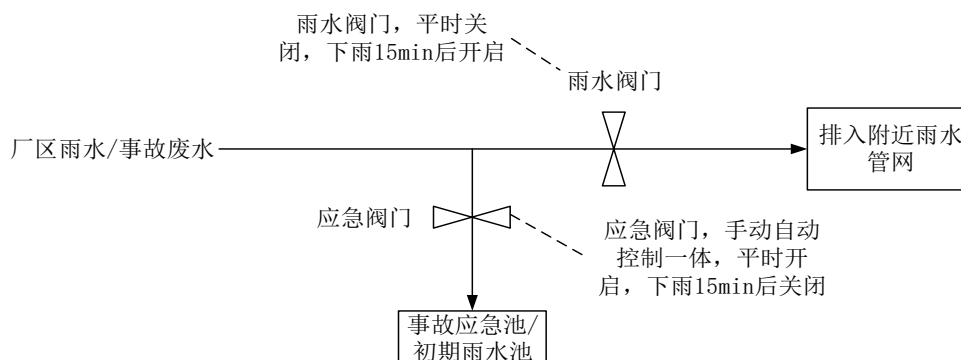
图 6-6 厂区事故废水（消防废水）收集系统示意图
