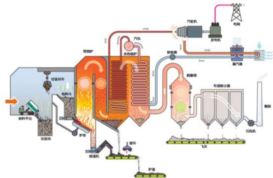
图 4-1 项目垃圾焚烧处理工艺流程示意图
