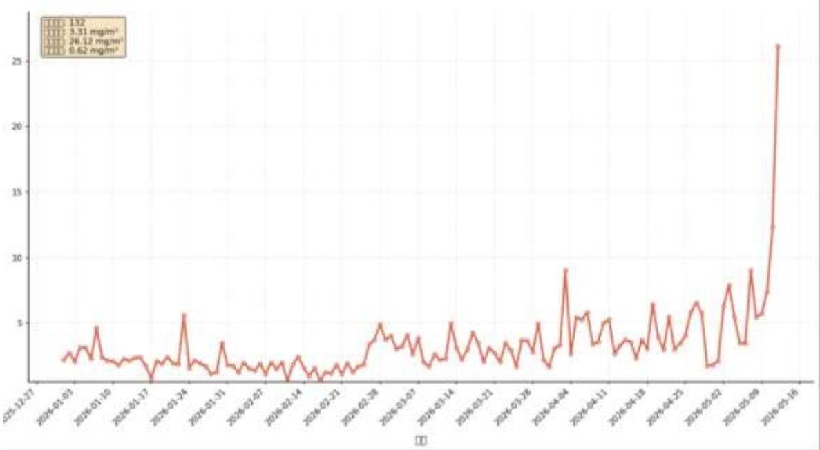
图 3-16 现有企业 2026 年上半年 3#炉一氧化碳在线检测数据图（日均值）
