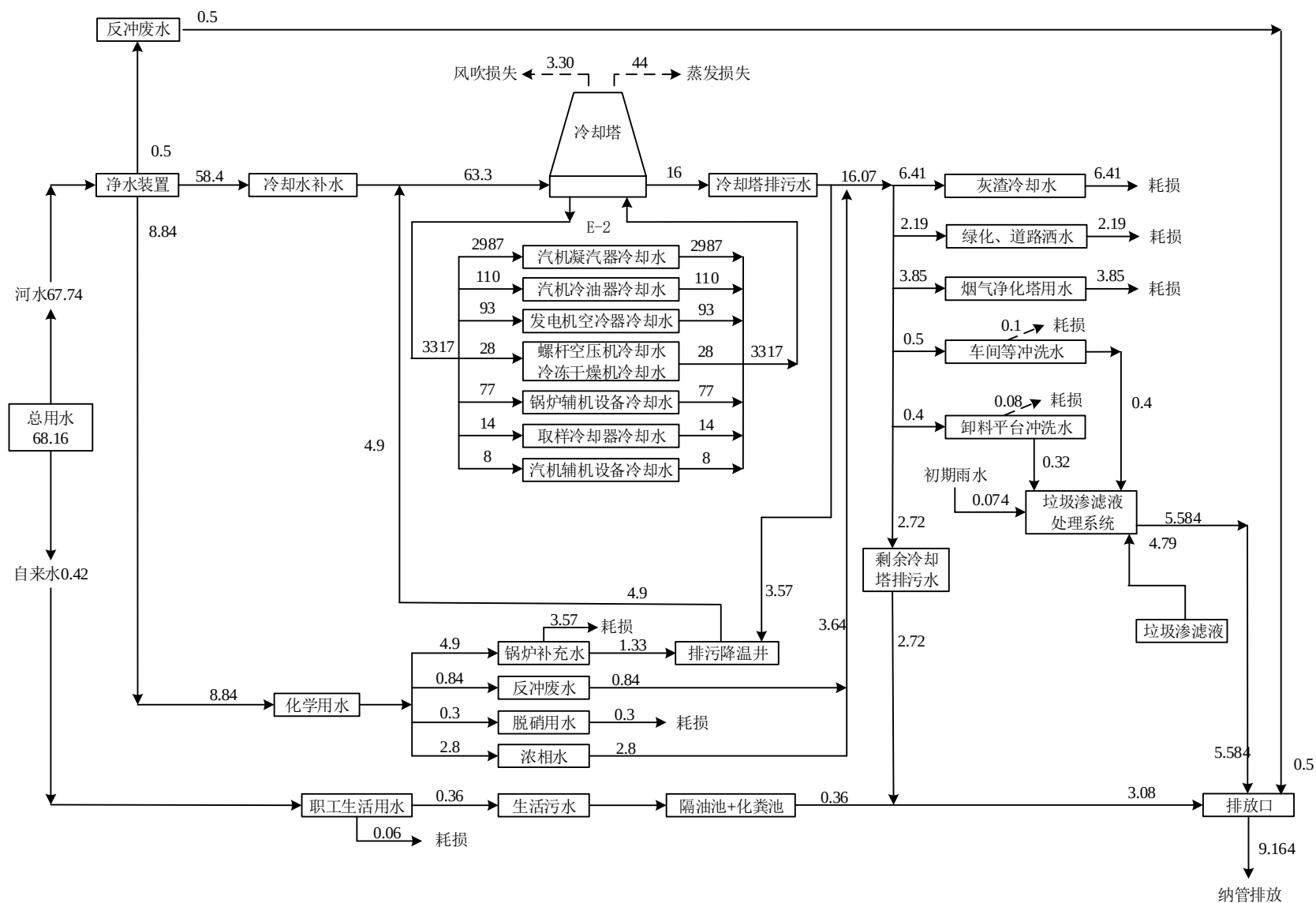
图 4-4 项目水平衡图 单位: t/h, 年工作时间 8000h/a
