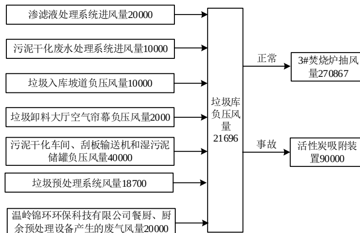
图 3-7 企业现状垃圾库内送排风量平衡图 单位: \text{m}^3/\text{h}
