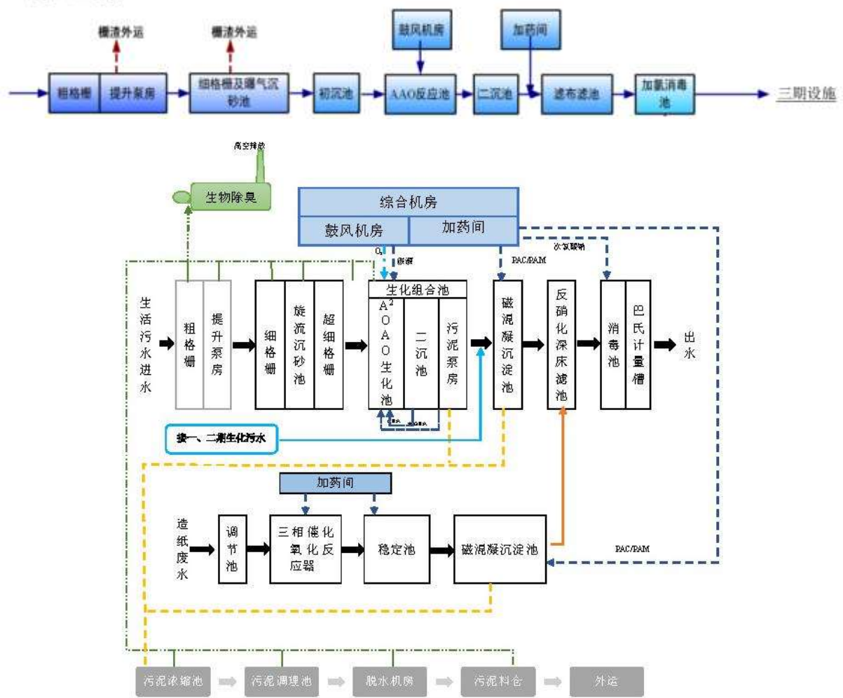
图 5-2 项目提标扩建后全厂污水处理工艺流程图
