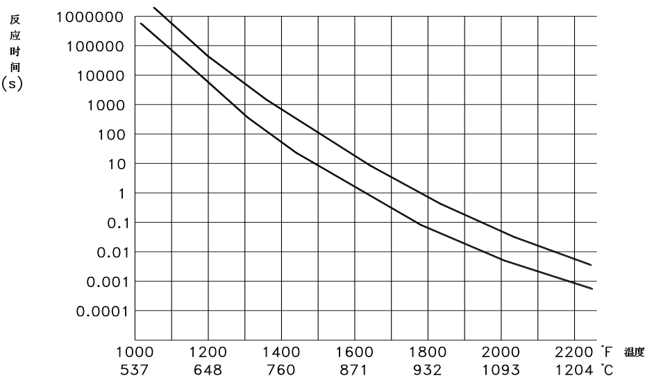
图 7-13 二噁英（TCDD）分解 99.99%所需时间
