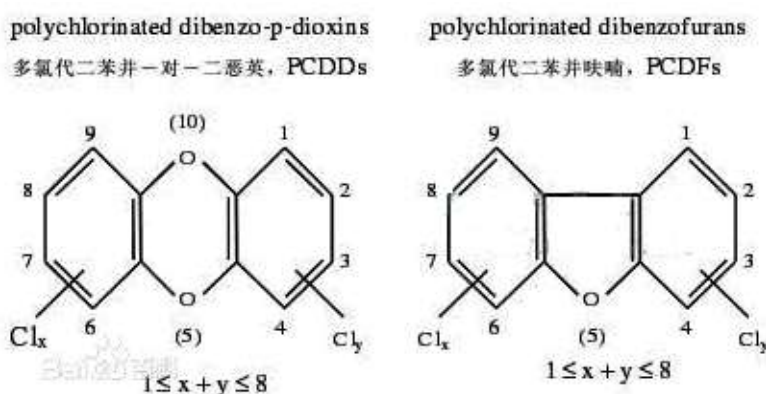
图 7-12 二噁英典型结构示意图
