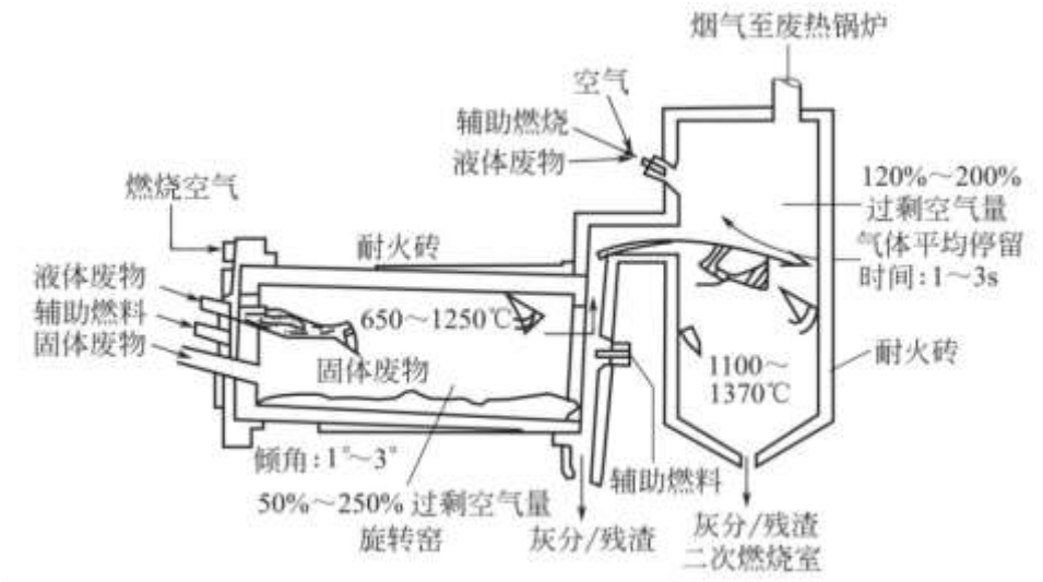
图 7-3 回转窑炉工作示意图
