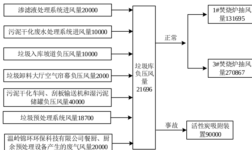
图 4-3 技改后垃圾库内送排风量平衡图 单位: \text{m}^3/\text{h}
