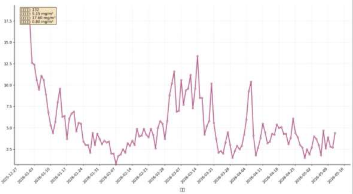
图 3-12 现有企业 2026 年上半年 3#炉二氧化硫在线检测数据图（日均值）
