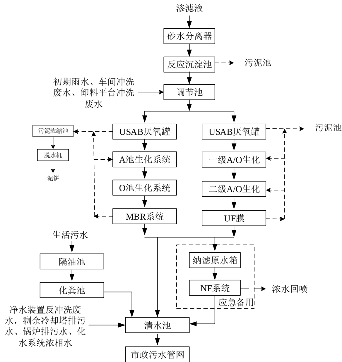
图 7-14 一期、二期项目污水处理设施流程图
