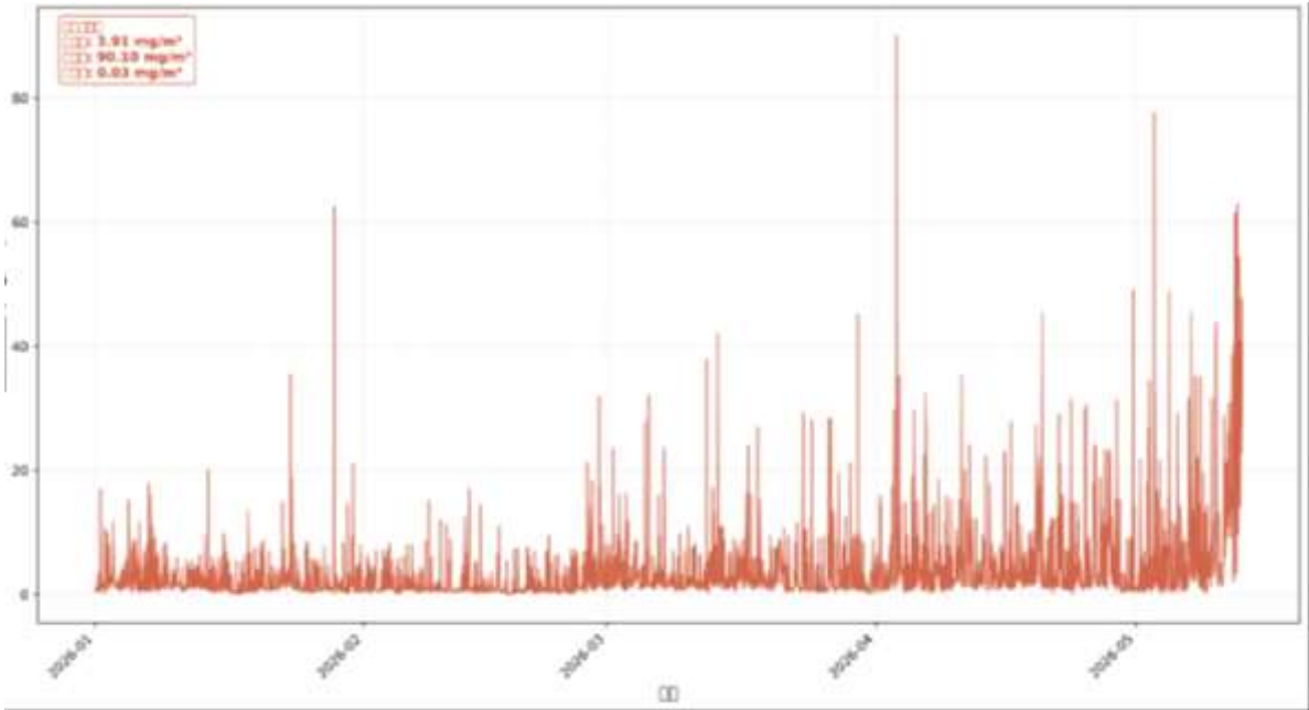
图 3-17 现有企业 2026 年上半年 3#炉一氧化碳在线检测数据图（小时值）
