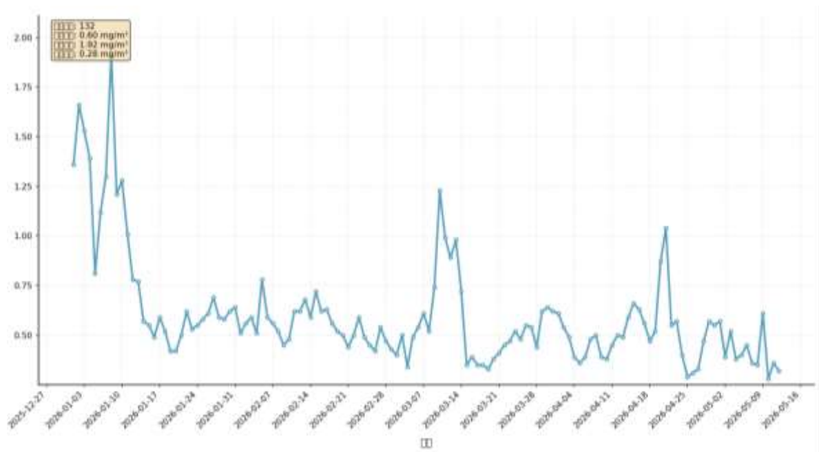
图 3-10 现有企业 2026 年上半年 3#炉颗粒物在线检测数据图（日均值）
