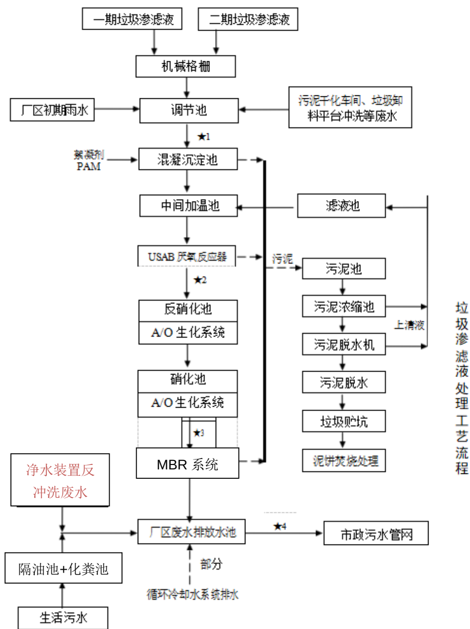
图 3-8 一期、二期项目污水处理设施流程图
