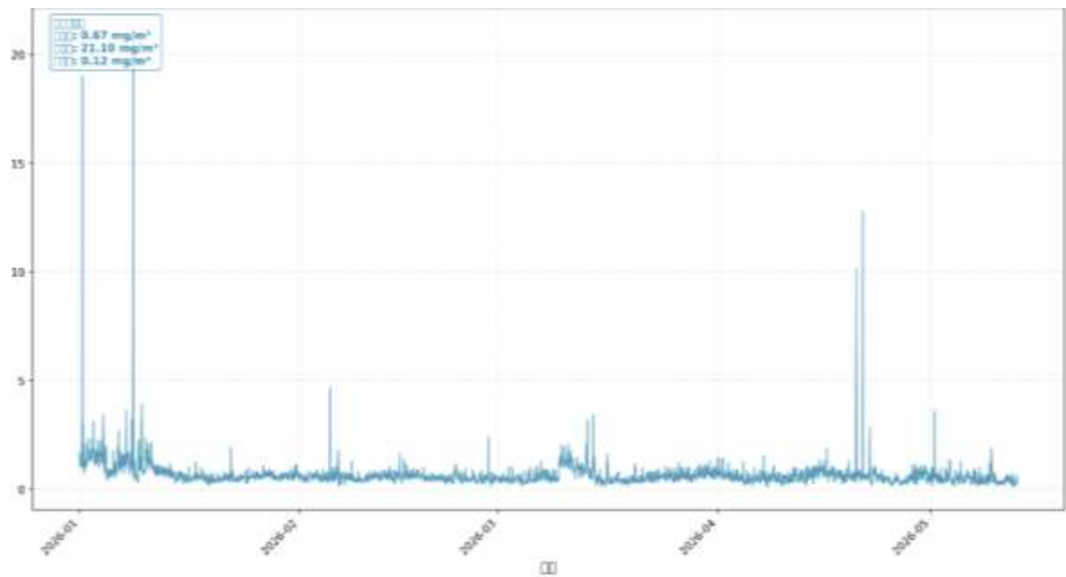
图 3-11 现有企业 2026 年上半年 3#炉颗粒物在线检测数据图（小时值）
