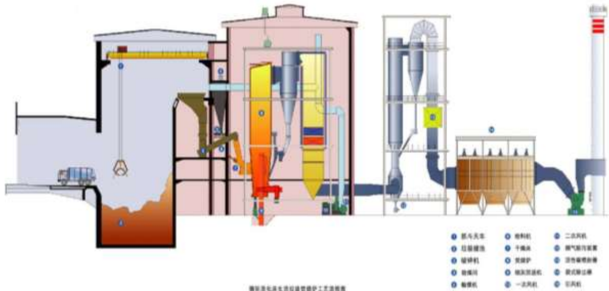
图 7-2 循环流化床焚烧炉工作示意图
