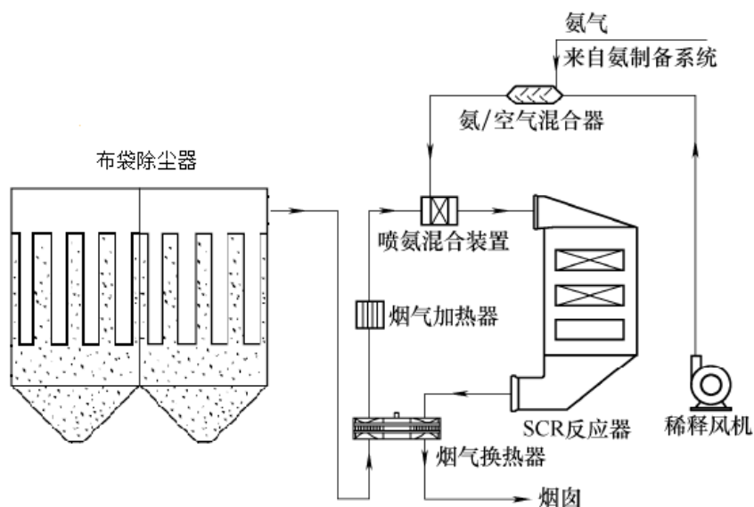
图 7-11 选择性催化还原法 (SCR) 工艺流程示意图
