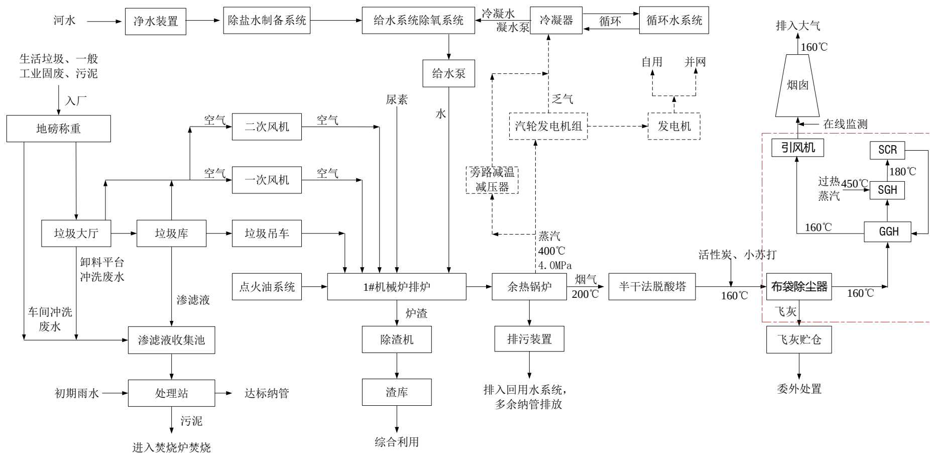
图 4-2 项目 1#炉生产工艺流程图
