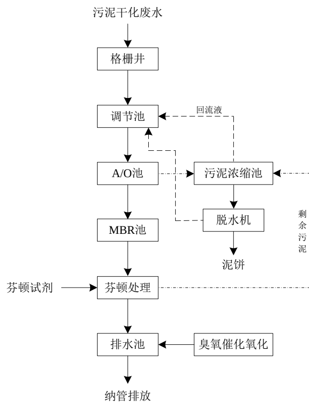
图 7-15 污泥干化项目污水处理设施流程图
