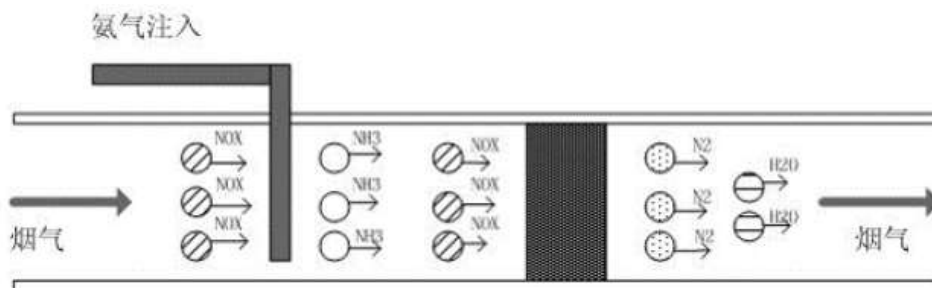
图 7-10 催化反应示意图
