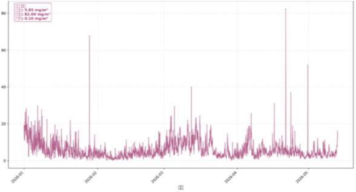
图 3-13 现有企业 2026 年上半年 3#炉二氧化硫在线检测数据图（小时值）
