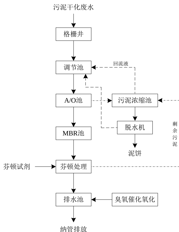
图 3-9 污泥干化项目污水处理设施流程图
